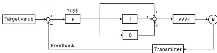
Фигура 6-14 Блокова диаграма на PID управление
