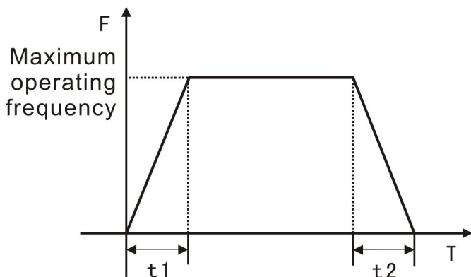
Фигура 6-1 Времеви криви на ускорение/забавяне
