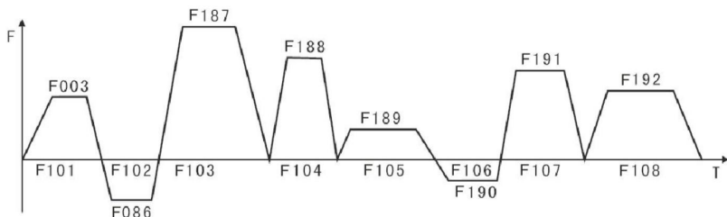
Фигура 6-9 Работна крива и контролни параметри за вътрешно контролирана многосегментна скорост [Описание] 1)
